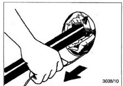
8.9 Füllschlauch in einem Zug in Kabelrichtung herausziehen.
